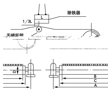
外形尺寸图
