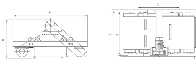
外形尺寸图
